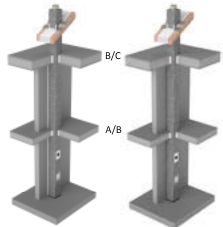
Bild 9: Abstände gemäß Bauartzulassung Z-7.4-3522
